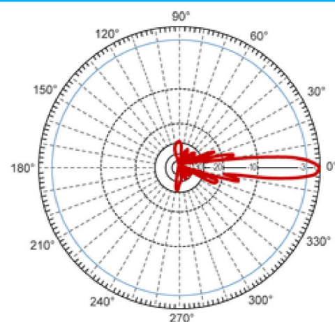
H-Plane
